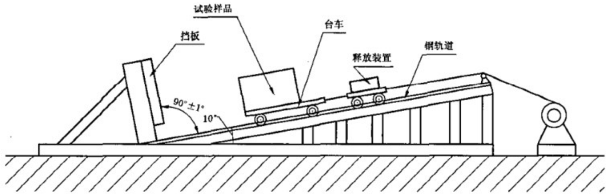
图 1 斜面冲击试验机简图
