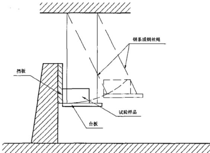
图 2 吊摆冲击试验机简图
