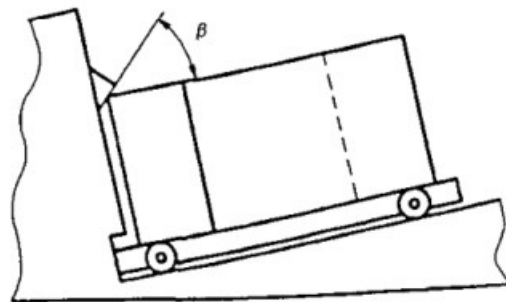
图 4 对一角的冲击, 试验样品的位置允许误差
